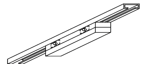
레일 콘센트용 플러그 및 이를 이용한 레일 콘센트용 조명기구 2015. 03
