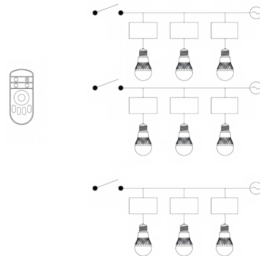
02. 무선 통신을 이용한 컨버터 모듈을 포함하는 조명 제어 시스템 2015. 01
